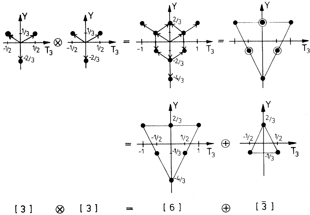
8. ábra: A [3] \otimes [3] ábrázolás megszerkesztése.
