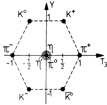
6. ábra: A J^P = 0^- pszeudoskalár mezonok.
