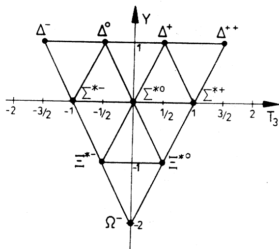
2. ábra: A J^\pi = \frac{3}{2}^+ barionok.
