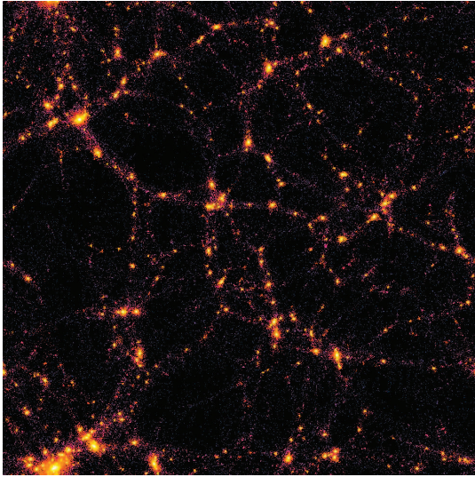
25. ábra. A buborékszerkezetet mutató világegyetem. Látható, hogy a csillagvárosok rendszerei mintha a nagy buborék belsejében lévő kisebb buborékok felszínén helyezkednének el.
