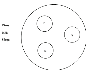
13. ábra. Protonban illetve neutronban három, egymástól különböző színtöltésű kvark fordul elő, ezért a proton és a neutron színtelen
