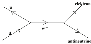
14. ábra. Neutron protonná való bomlásakor a neutron belsejében egy d kvark u kvarkká alakul át. Eközben egy virtuális W^- bozon keletkezik, amely elektronná és antineutrinnóvá bomlik.
