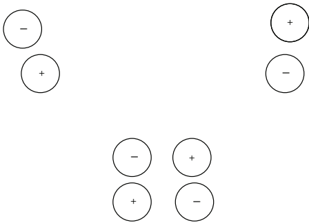
1. ábra. Van der Waals erő. Ha két hidrogén atom egymás közelében kerül, az elektronok térbeli eloszlása kismértékben csökkenti a két proton közötti taszítást
